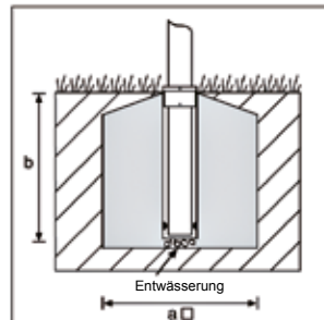
Zentrierhülse: Standard für Ø 100 mm, NH 7/8/9 m
