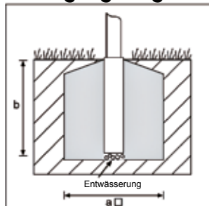
Passform-Bodenhülse: Standard für Ø 90 mm, NH 6/7/8 m
